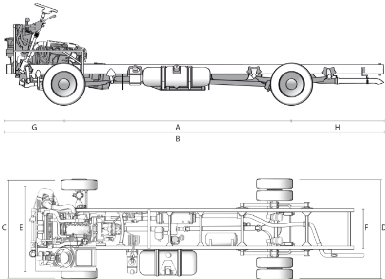
CHASSI MA 9.2
